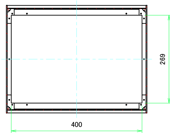
B-B ( 1 : 6 )
