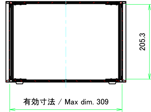
A-A ( 1 : 6 )
